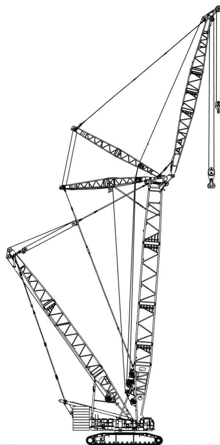
HL-ラフティングジブ
