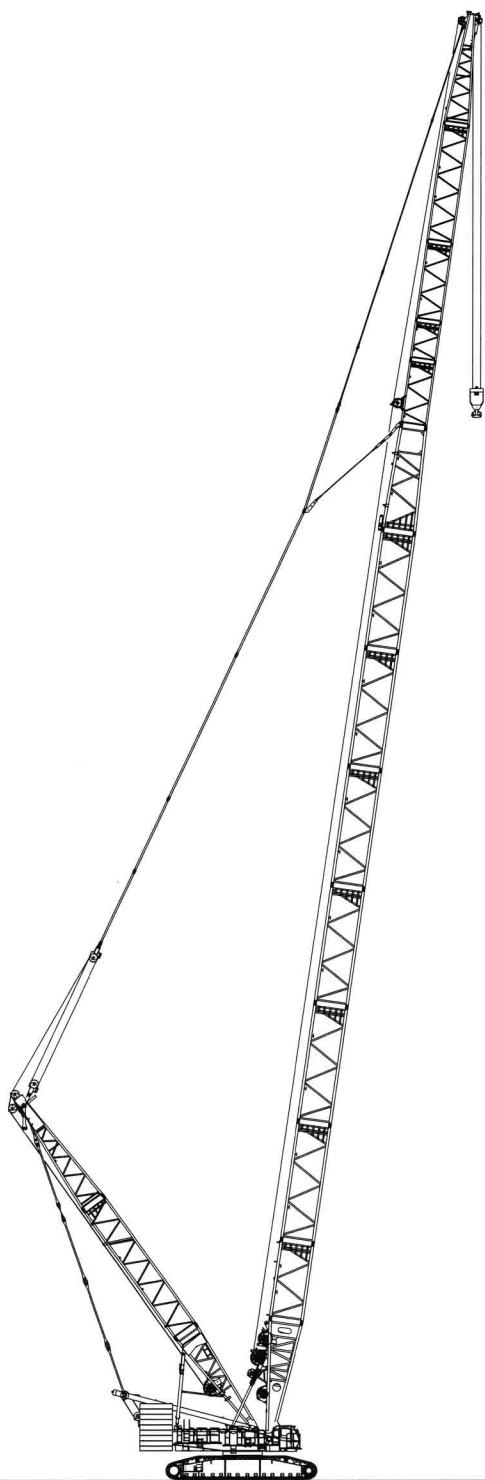
HL-ロングブーム
