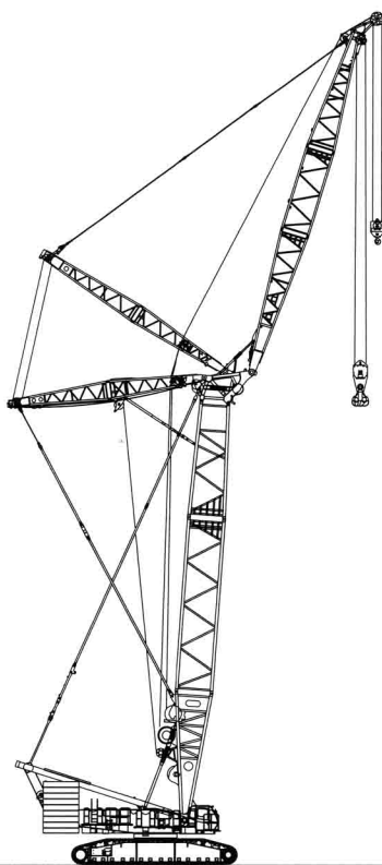
STD-ラフティングジブ
