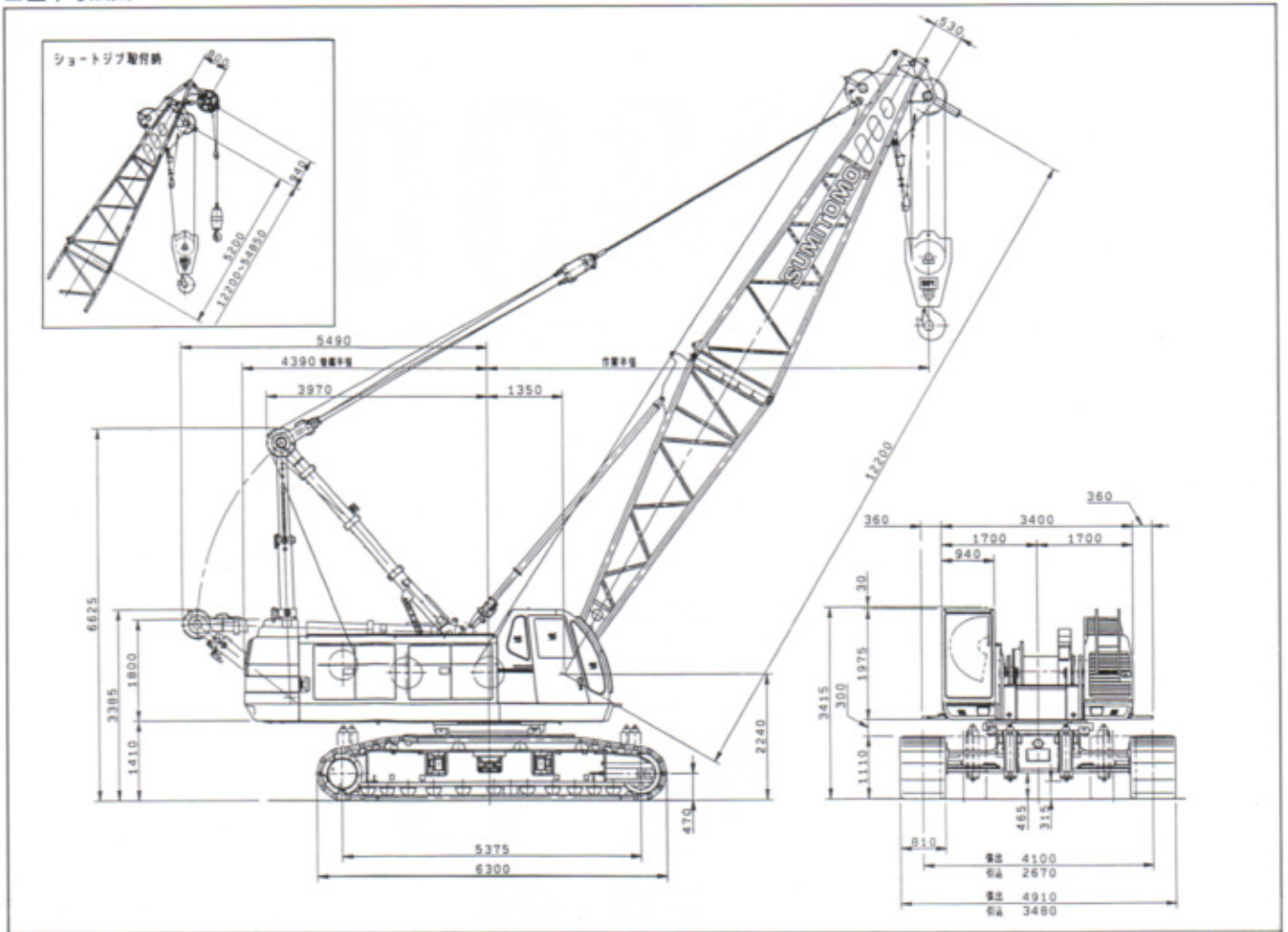
■基本寸法図
