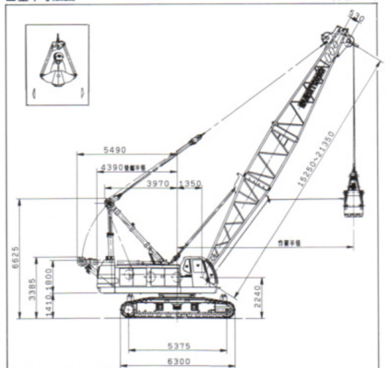
■基本寸法図
