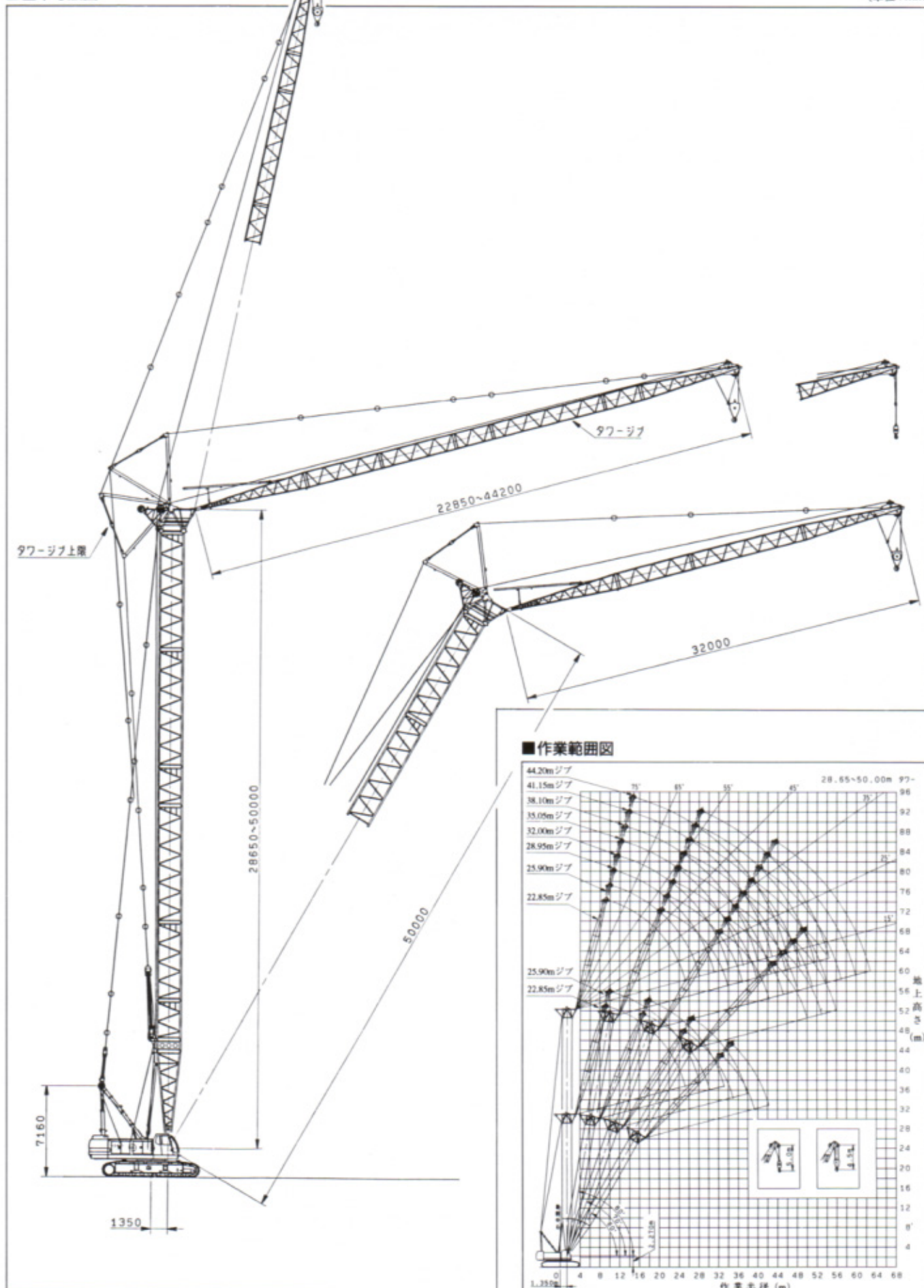
■基本寸法図
