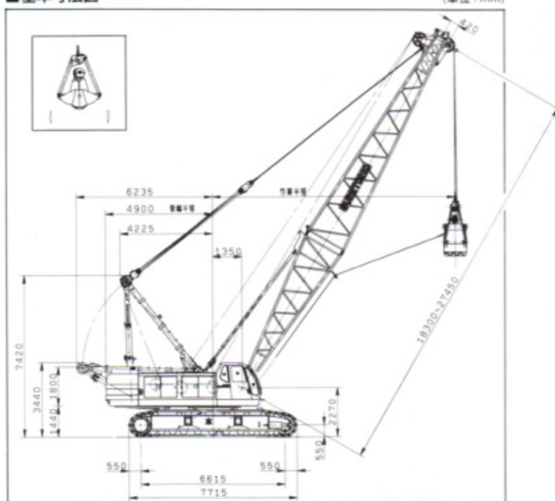
■基本寸法図
