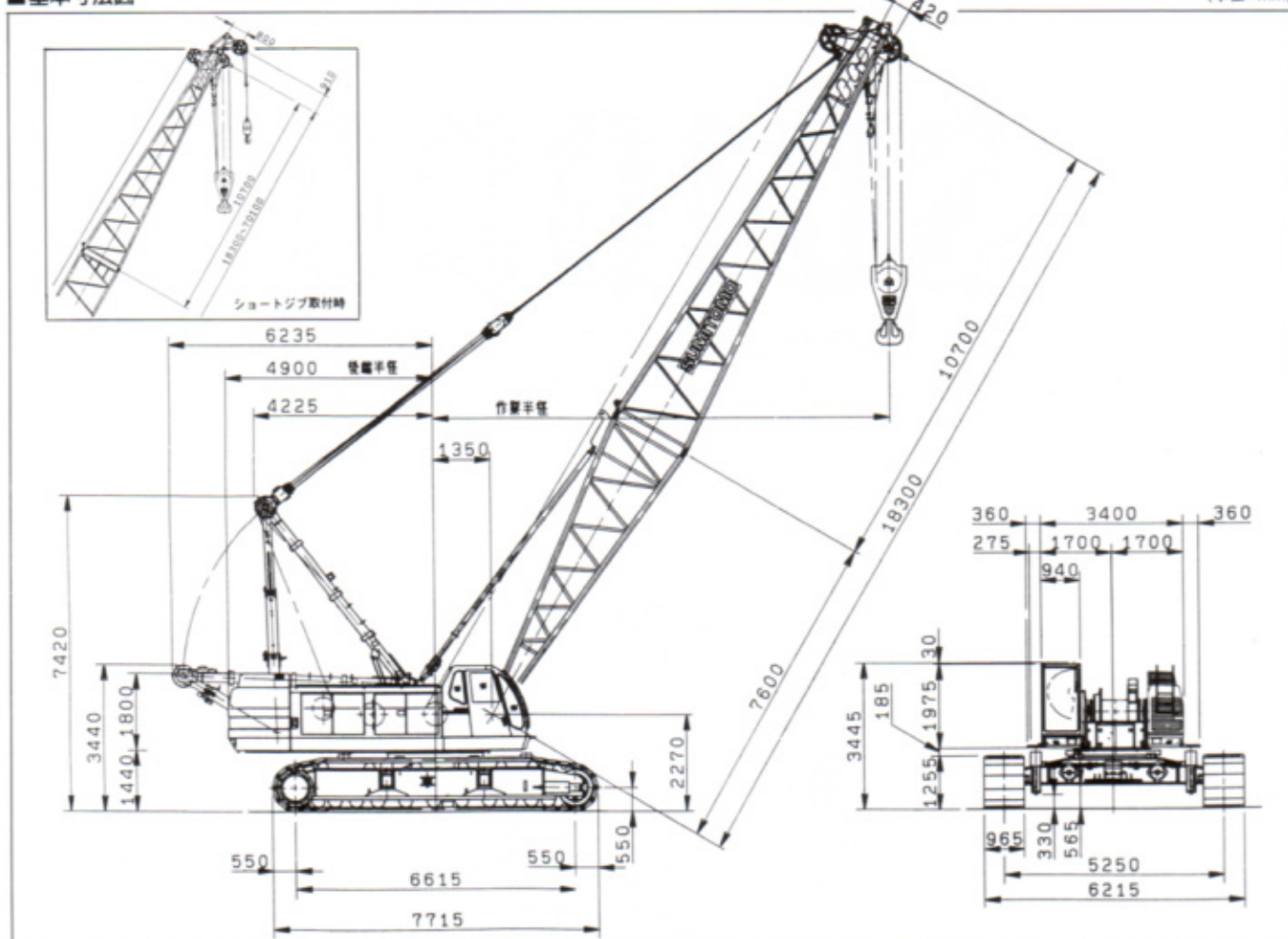
■基本寸法図
